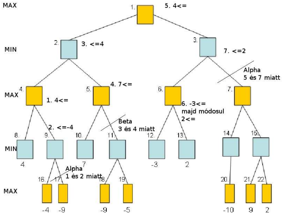
Az 1. ábrán látható egy Min-Max feladat teljes megoldása Alpha-Beta vágás használatával.
