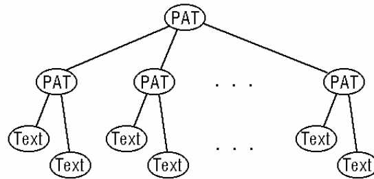
19. ábra. Az örkeresztek adatait tartalmazó DG-adatstruktúra
