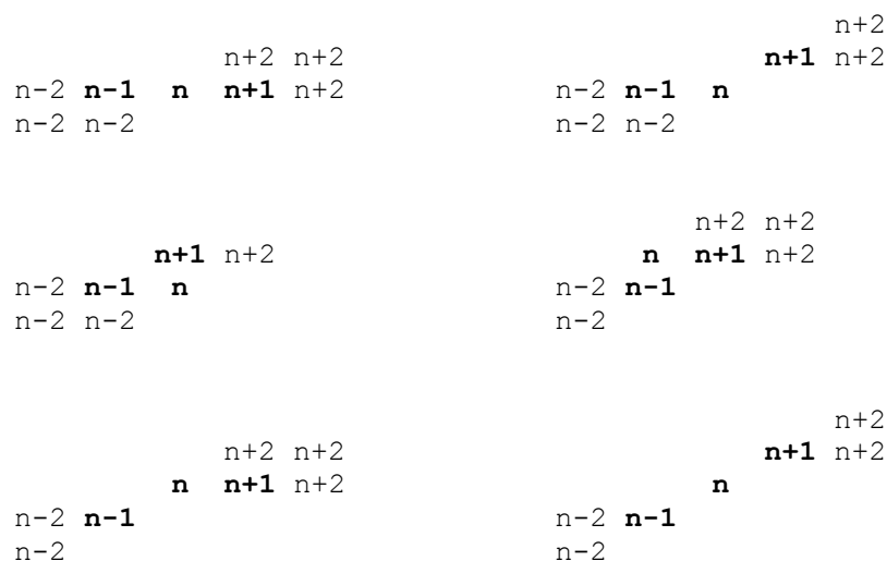
60. ábra. Lehetséges esetek a 2. állítás bizonyításához.
