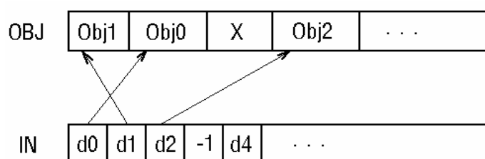
13. ábra. Az Obj és In tömbök kapcsolata. Az X egy törölt objektum helyét, -1 a rá való hivatkozás helyét jelöli
