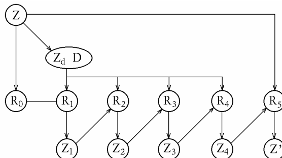
51. ábra. Multigrid eljárás vázlata n = 5 esetén. Z_d és D magyarázatát lásd később
