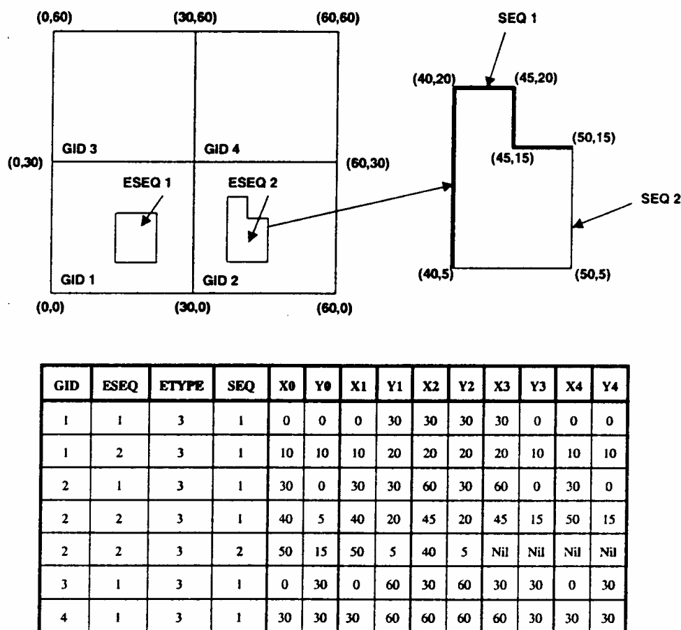
10. ábra. Az OpenGIS (1997) által adott példa poligonok tárolására relációs adattáblában
