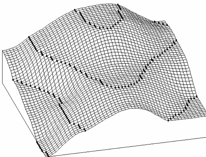
53. ábra. Egyszerű redukciós eljárással nyert DTM. A teraszhatás érzékelhető
